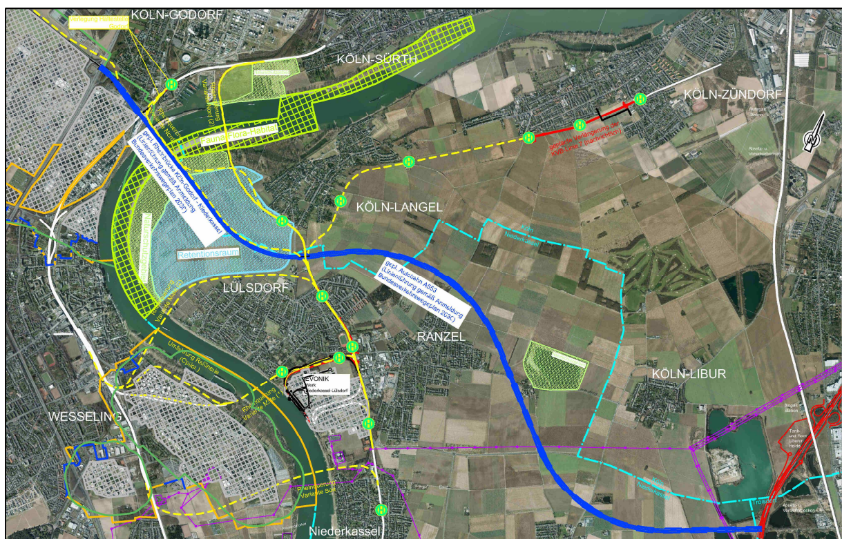
Abbildung 9: Varianten der Rheinbrücke (Vorzugstrasse: durchgezogene gelbe Linie)
