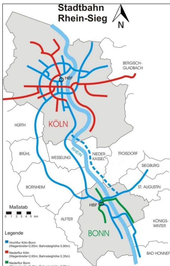
Ausbaup Option 1 mit Anschluss an Linie 17 Integration in das Hochflursystem Köln - Bonn
