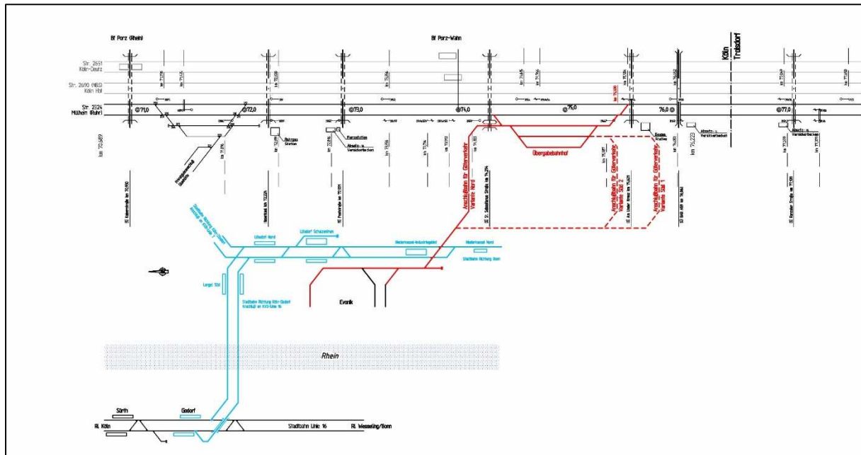
Abbildung 10: Einbindung der Güteranschlussbahn (Varianten 1 bis 3) in das Schienennetz
