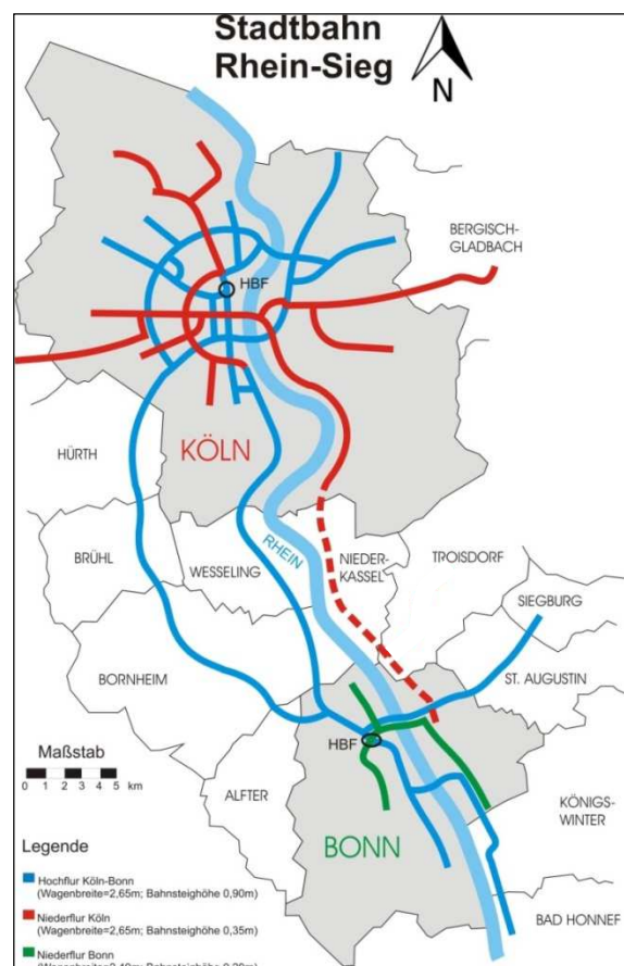
Ausbaup Option 2 mit Anschluss an Linie 7 Integration in das Niederflursystem der KVB
